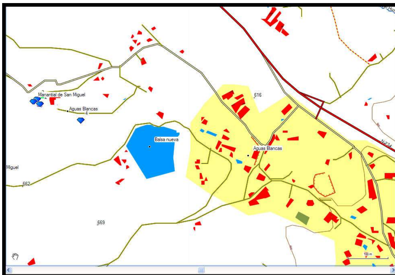
Detalle de situación de los cuatro afloramientos de San Miguel
